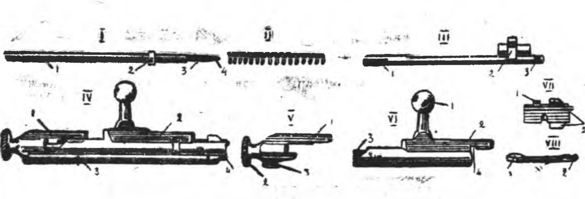
I. Уларник 1. Гол 2. Бэлхэй 3. Лопасть 4. Сооалуур II. Дайшалхы пружина III. Хабсаргаша планка 1. Нюрган 2. Тулга 3. Сосок IV. Затвор 1. Курок 2. Затворой шалбэ 3. Хабсаргаша планка 4. Дайшалхы личинкэ V. Курок 1. Нюрган 2. Пуговка 3. Дайшалхы лэгэ VI. Затворой шалбэ 1. Барюул 2. Нюрган 3. Шурбэтан отолборн 4. Хабсаргаша планкын тулгын нюрганай дай.
