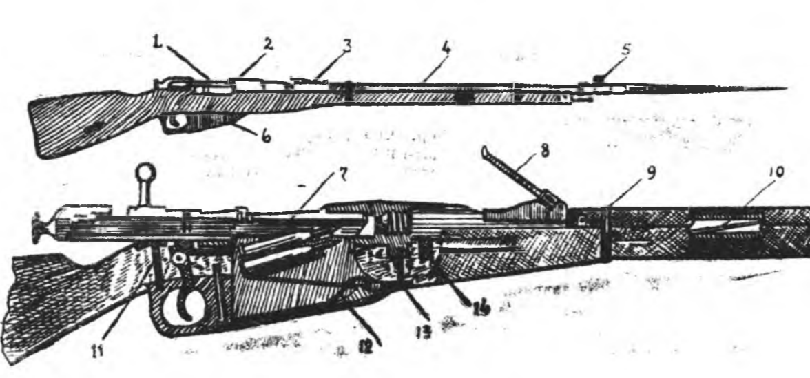
1. Затвор 2. Сэмгэнэй коробко 3. Хойто харагай колдоко 4. Сэмгэнэй хабхаг 5. Уриа хараа халхашатаа 6. Магазинна коробко 7. Сэмгэнэй коробко 8. Харагай рамка 9. Шалбын сахариг 10. Хэршэлээ 11. Шалбын зууурай шүрбэ 12. Үргэх оньшон 13. Тулга шүрбэ 14. Шомполой тулга
