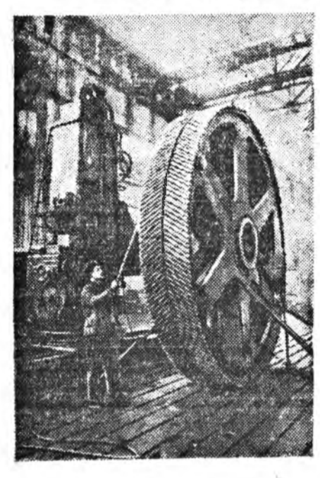
ДОНБАСС. Сталиний нэрэмжэтэ Номо-Браморо заводой № 1 механичска цехын строгальник станционер М. И. Павлов шайншэ подъемно машинада зургаан метр диаметрий сахарт дархалан бүтээжэ байба. (ТАСС-эй фотохрошкю).
