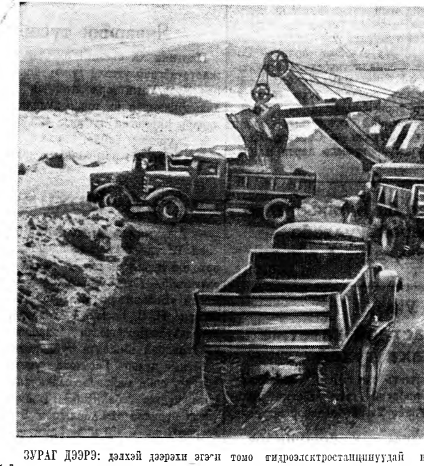
ЗУРАГ ДЭЭРЭ: дэлхэй дээрхи эгэни томо гидроэлектростанцинуудай пазни болохо Братска ГЭС-эй барилга ахилжа байна. М. МИГ_ФВЗЙ фото.
