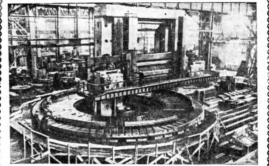
Московско область. Томо стапогуудые бүтээдэг Коломенско завод «КУ-16» маркын томо станок бүтээн гаргаба. Энэ станок турбинануудай 260 тонно хүрэтэр гэгшүүртэй мөөрнүүдые мүлүн залхаха юм.
