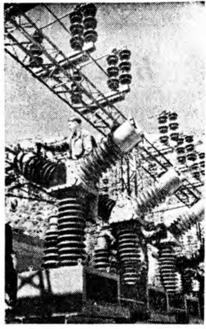
Грузинска ССР. Ткубилска ГЭС-эй барилга дээрэ нэмэл подстанци хабсаргагдажа байна. ЗУРАГ ДЭЭРЭ: подстанцие хабсаруулаха харуулагдана. ТАСС-эй фотохронико.
