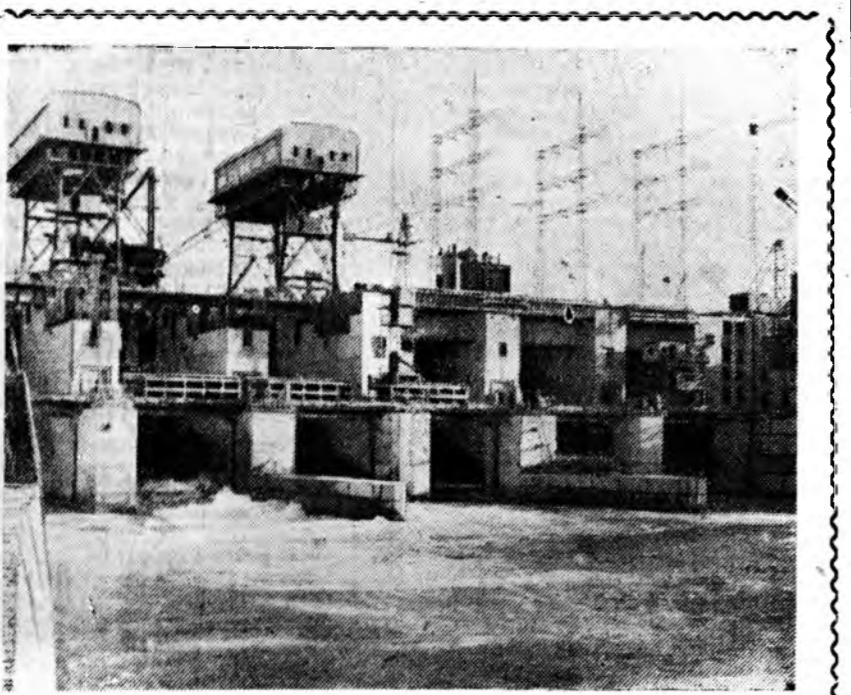
ТАДЖИКСКА ССР. Кайрак-Кумска ГЭС-тэ түрүүшын агрегат хабар-гагалажа, туршагдһан шагдагдаба. Мүнөө хоёрдох турбинаны табигдажа байна. ЗУРАГ ДЭЭРЭ: Кайрак-Кумска ГЭС-эй гидроузел. ТАСС-эй фотохүснэгт о.
