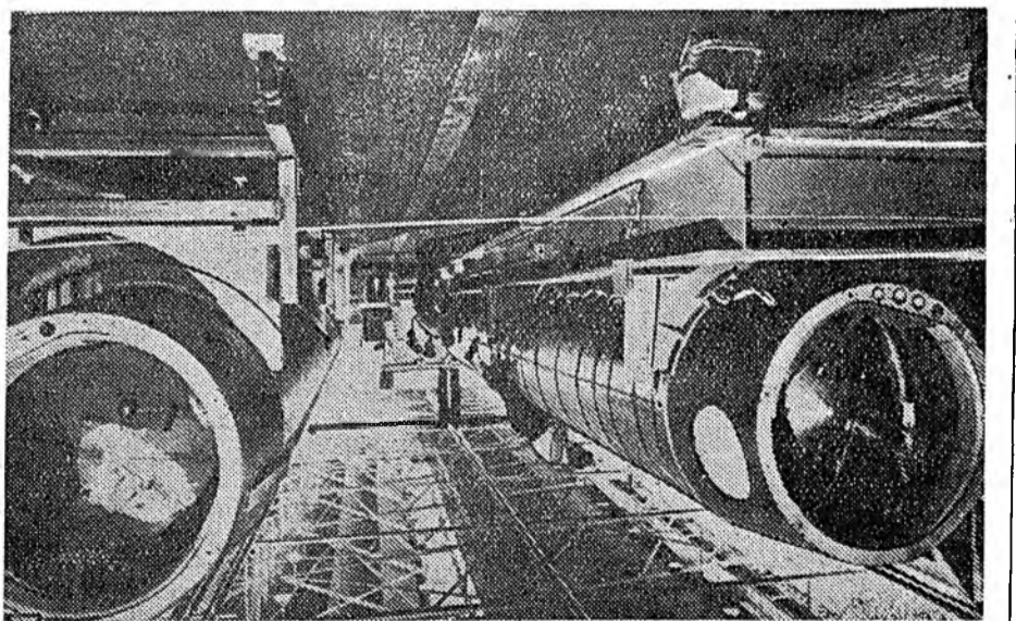
Газар дэлхэйтэй зэргэсэн дабшаха ракетэ табиһын тула. Америкын Холбоото Штадууд бэлдэжэ байна. Дөһөндэ дэгдэхэһэн тула гурбан самсаалтай томо ракетэ бүтээжэ гэжэ багсаагдана. Тэрэн эрхэ жэлдэ бэлэн бодохо юм ха. ЗУРАГ ДЭЭРЭ: тиймэ ракетын бүтээгдэжэ байһан Балтимортохи заводой цех дотор. ТАСС-эй фотохронико.
