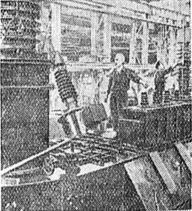
Запорожье. Трансформаторна заводой хүдэлмэрилэгшэд шэнэ трансформаторнууды бүтээгэд болжо байна. Хабаралтын цехтэ 90 мянган киловатт-ампер хүсэтэй, 400 киловольт хүсэтэй автотрансформатор бүтээгдэб. ЗУРАГ ДЭЭРЭ: шэнэ автотрансформатор туршагдаһан. ТАСС-эй фотохронико.
