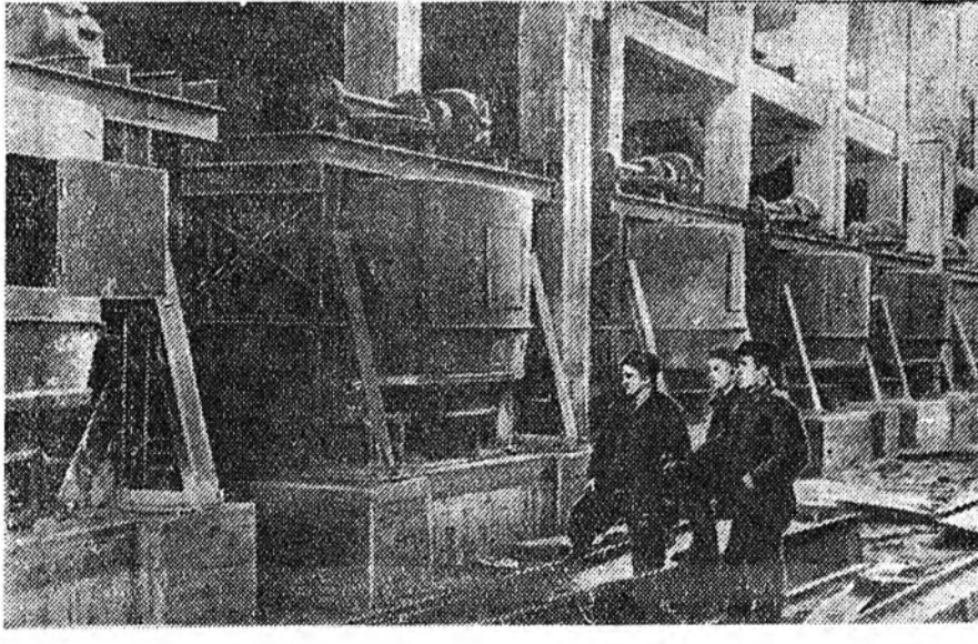
ЗУРАГ ДЭЭРЭ: Темлюйска шиферэй заводой барилганад гол корпус соо «бегуны» гэжэ машинануудыс тодохжо дүүргэд байна.
