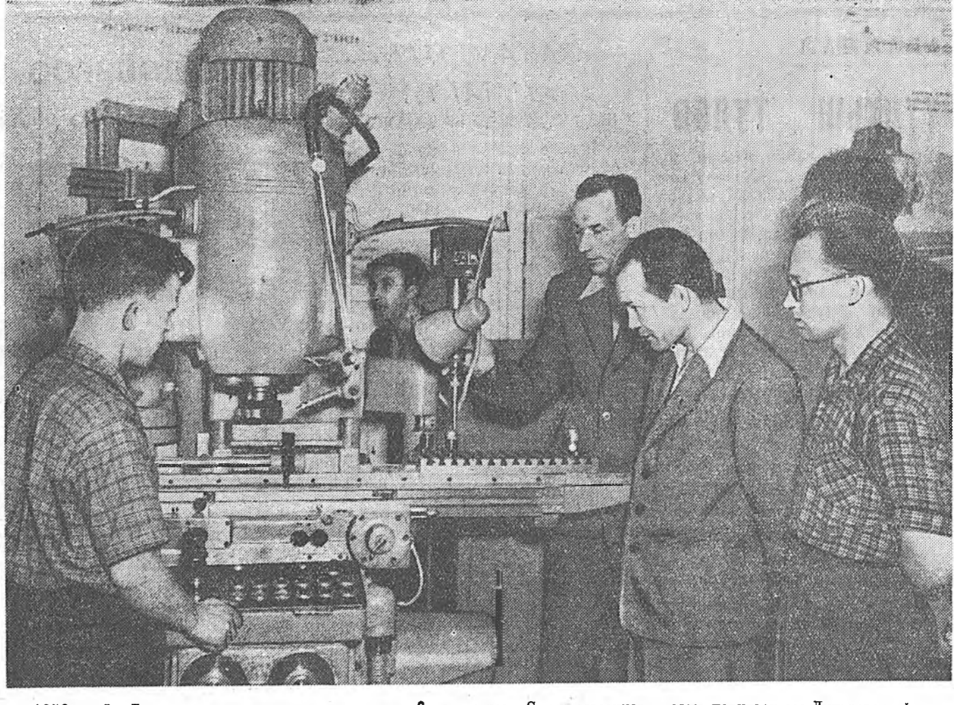
1958 оной Бүхэсоюзна промышленна выставка. Зураг дээрэ: «Станкостроение» гэжэ павильон соо Дмитровско фрезерная станок бүтээдэг заводой хүдэлмэришлэл А. Кудряшев заводойгоо бүтээһэн станок тухай выставкда орошодто харуулжа байна.
