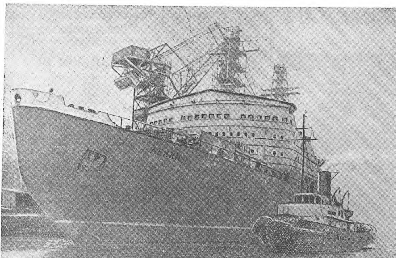
Ленинград. Советскэ Союзда баригдажа байһан түрүүшнэй атомна корабль, дэлхэй дээрхи эгээн томо «Ленин» гэжэ атомна ледокол туршагдажа байһай. Корабль бүтээгшэд тэрэнэй олон тоото машина, механизм, прибор болон атоматическа түхээрал, энүүдыг шалган үзэжэ байһай. Зураг дээрэ: «Ленин» ледокол заводой дэргэдэ байна.
