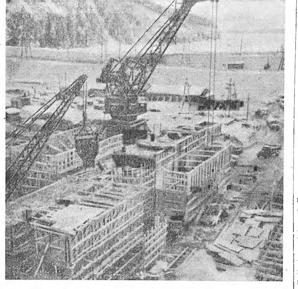
Братск ГЭС-эй барилга дээрэ. 1961 ондо энэ ГЭС-эй түрүүшын хубине ашагдалга оруулхын түлөө барилгад тэмсэнэ. ТАСС-эй фотохронико.
