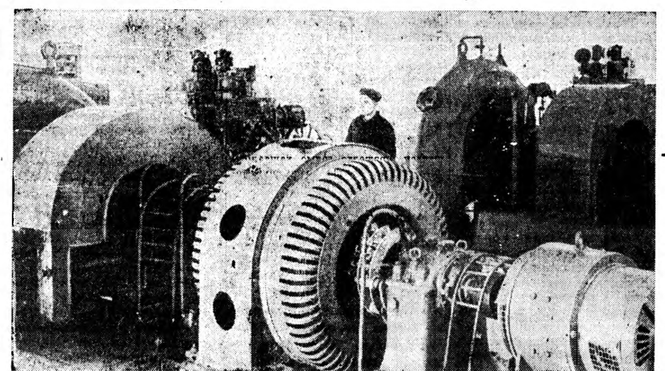
Эндэ колхоз хоорондын хэднэ гидроэлектростанцинууд бии юм. Саашада Нестериха голдо найнаар ашаглахын тула мүнөө эндэ станцинууд хоорондоо холбогдожо, нэгдэмэл электросеть баригдажа байна. Зураг дээрэ: Курумжаны ГЭС-эй машинна зал собо.
