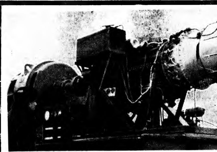
МОСКВА. Ная болот авиационно турбонитой двигателюуд агаарта ашагларда болзорой дүүрэхэдэ миң хангадаг байгаа. Мүнөө тэрэ двигателюуд теплогенераторууд болгондон хууле ажыхда орооно, кукуруза, хлопок хатаалга дээрэ үргэнөөр хэрэглэгдэнэ. ВУРАГ ДЭЭРЭ: энергоагрегат болгондон авиационно мотор.
