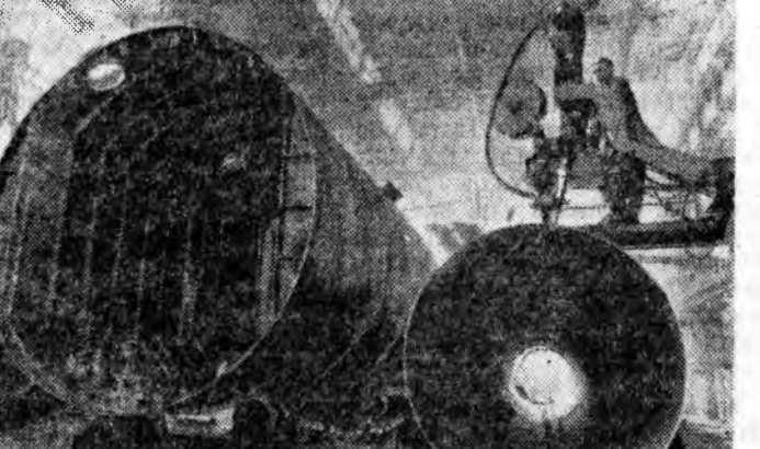
Брнодохи (Морави) Краловопольско машина бүтэглэги завод Братиславадхи «Словнафт» гэжэ химическа комбинатад хэрэгтэй атмосфера коллоннуудые бүтээн гаргадаг. Энэ хадаа Чехословакиа бүтэгдэдэг эгзэн лэ томо коллоно болоно. Тэрэнэй диаметр 5,5 метр, үндэринь 38 метр, шгүүнүүрш 233 тонно юм. Зураг дээрэ: коллоно хабсаргагдахар бэлтгэхэдэ.
