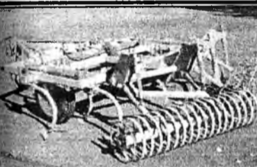
КУЛЬТИВАТОР КПЭ-3,8М с катками выравнивателями КВ-4
